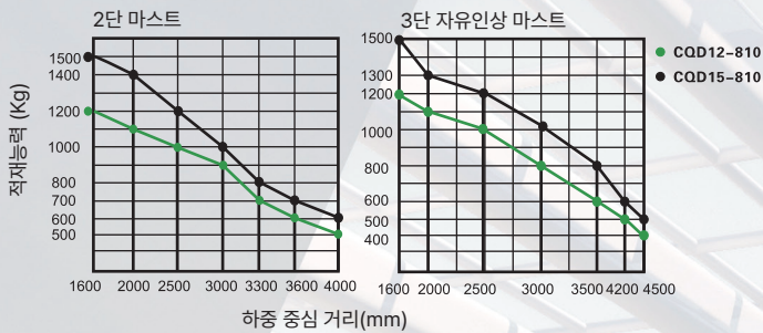
하중 곡선도
